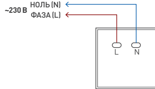
Рис. 1. Схема подключения
