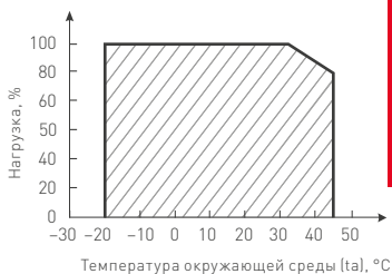
Рис. 3. Максимальная допустимая нагрузка, % от мощности источника
