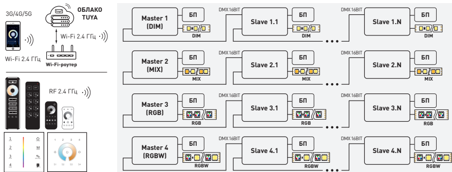
Рис. 2. Общая структурная схема построения системы управления освещением
