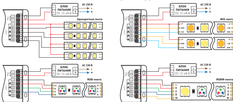
Рис. 4. Подключение источника питания и светодиодной ленты
