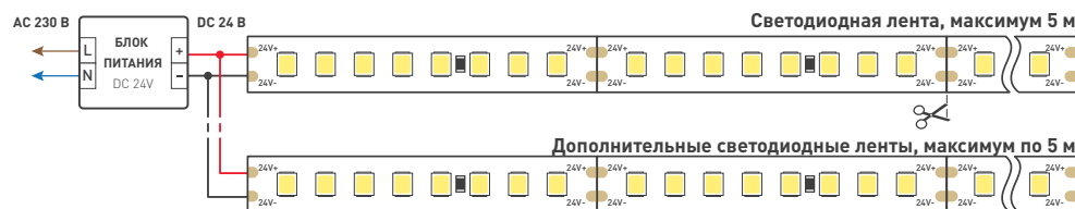
Рис. 1. Подключение нескольких светодиодных лент с одной стороны
