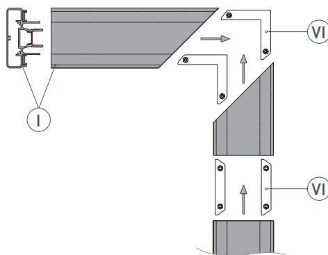
Рис. 1. Виды соединений
