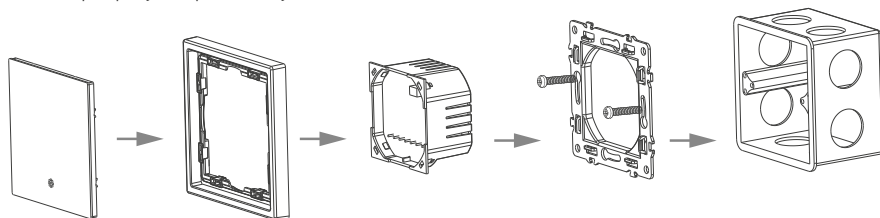
Рис. 3. Монтаж терморегулятора
