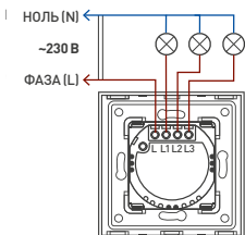
Рис. 3. Схема подключения (0500042,0500048,0500047,0500046)
