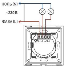
Рис. 2. Схема подключения (0500041,0500038,0500039,0500040)
