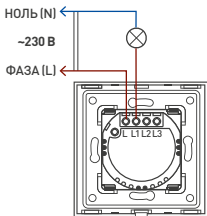
Рис. 1. Схема подключения (0500035,0500037,0500036,0500033)
